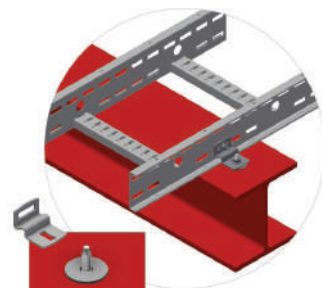
Soporte de bandejas y escalerillas eléctricas
